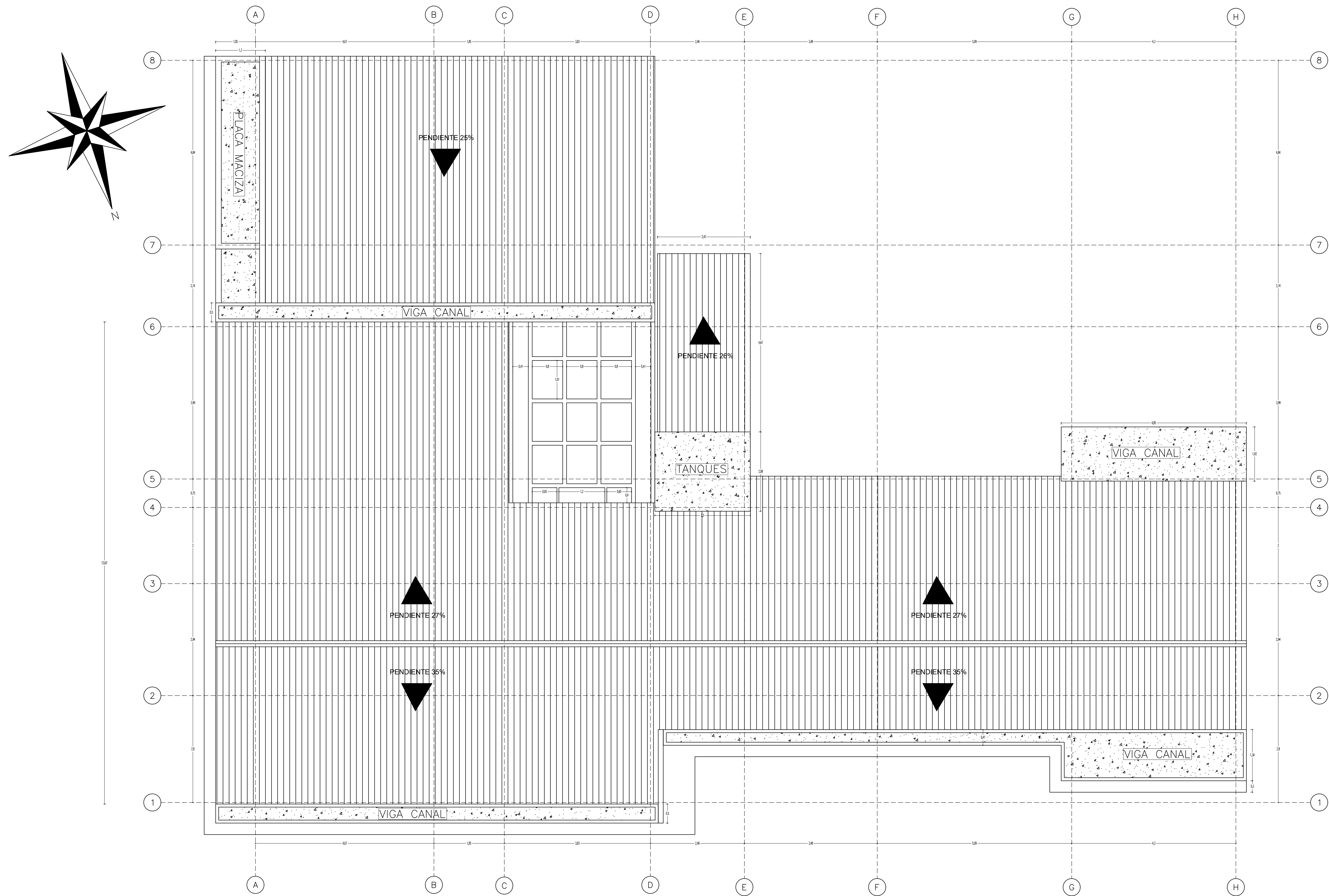
PLANTA CUBIERTA ESCALA 1:50
