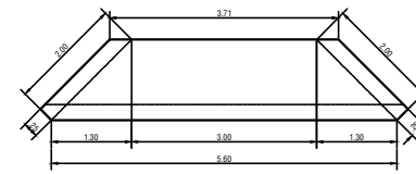
DIMENSIONAMIENTO SOLERA ESCALA 1:50
