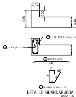
DETALLE GUARDARUEDA ESCALA 1:25
