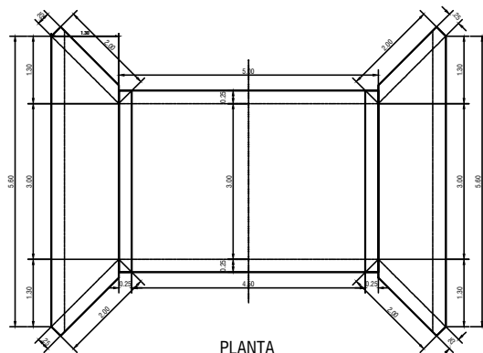
PLANTA ESCALA 1:50
