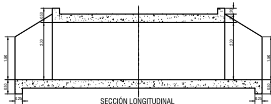
SECCIÓN LONGITUDINAL ESCALA 1:50
